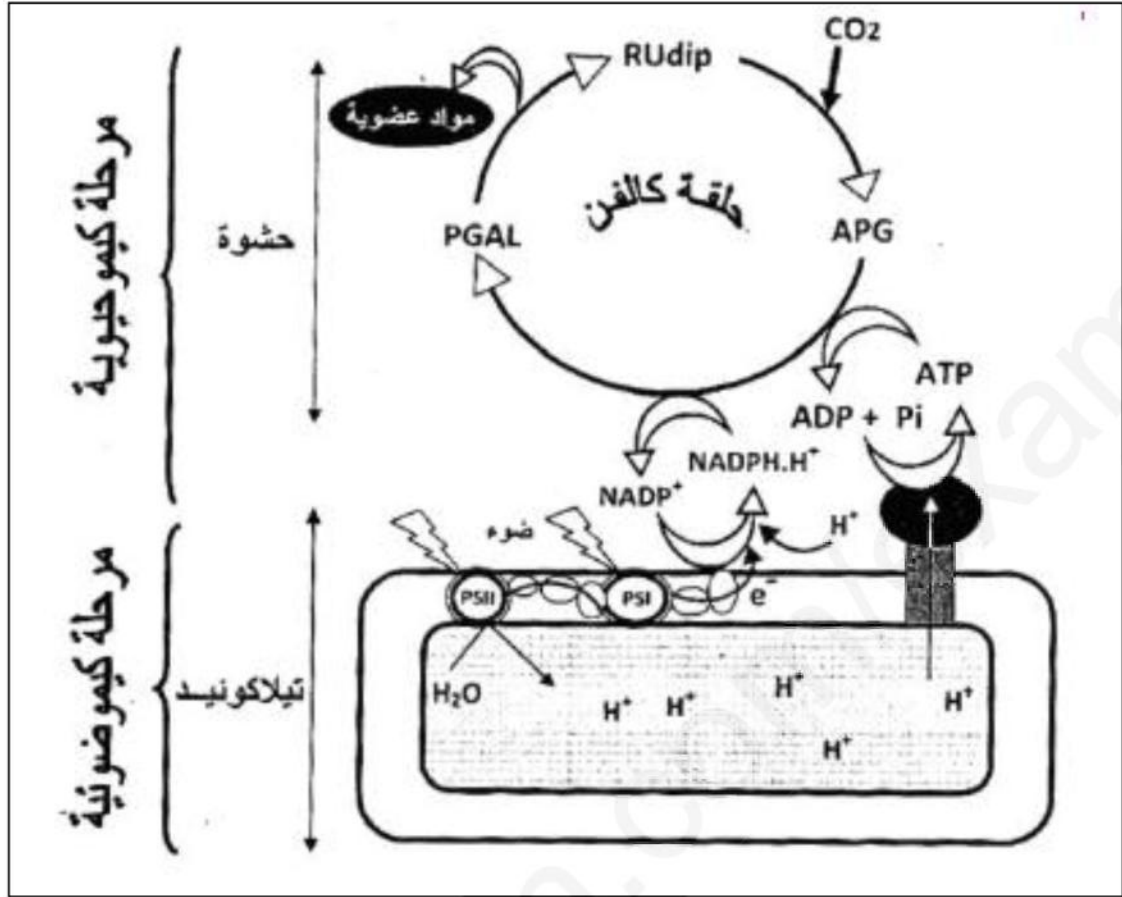
رسم تخطيطي يوضح التكامل بين مرحلتي التركيب الضوئي
